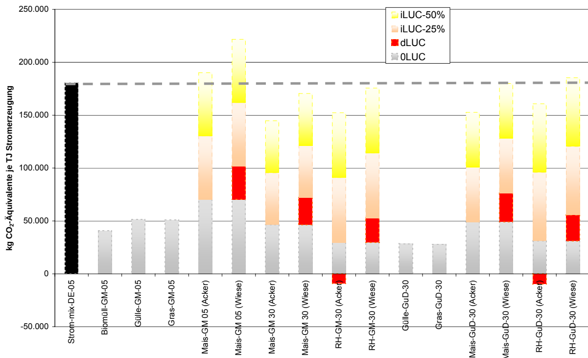
Bild 8 THG-Emissionen der Stromerzeugung aus Biomethan (Einspeisung)
