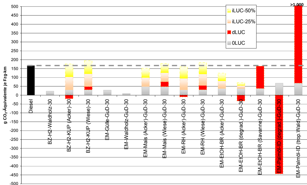
Bild 20 Verkehrsleistungsbezogene THG-Emissionen für BioGH 2 und biogenem Fahrstrom
