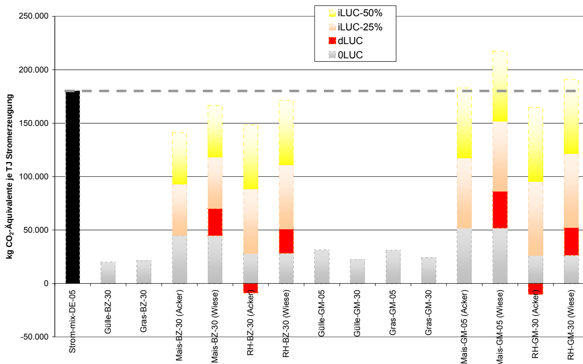
Bild 7 THG-Emissionen der Stromerzeugung aus Biogas (direkte Nutzung)
