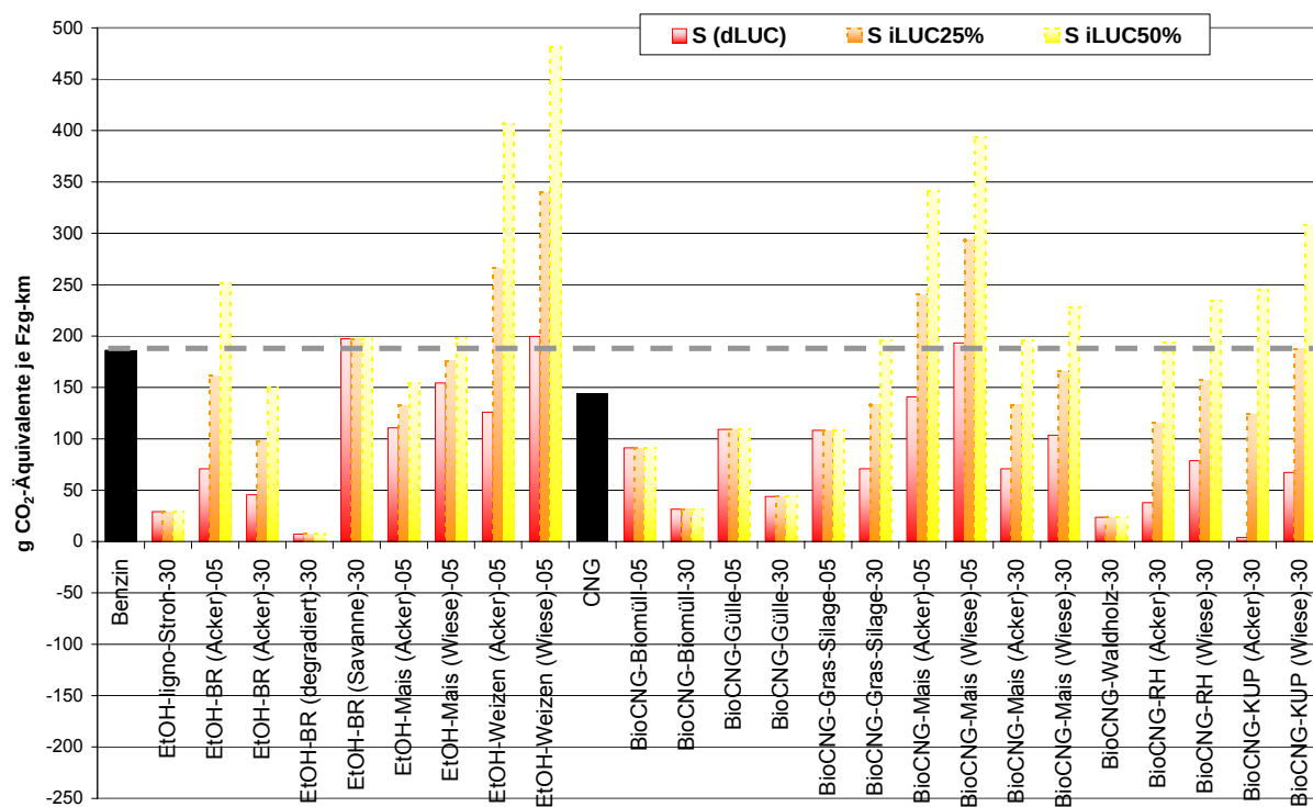
Bild 24 Kumulierte verkehrsleistungsbezogene THG-Emissionen für Bioethanol und BioCNG
