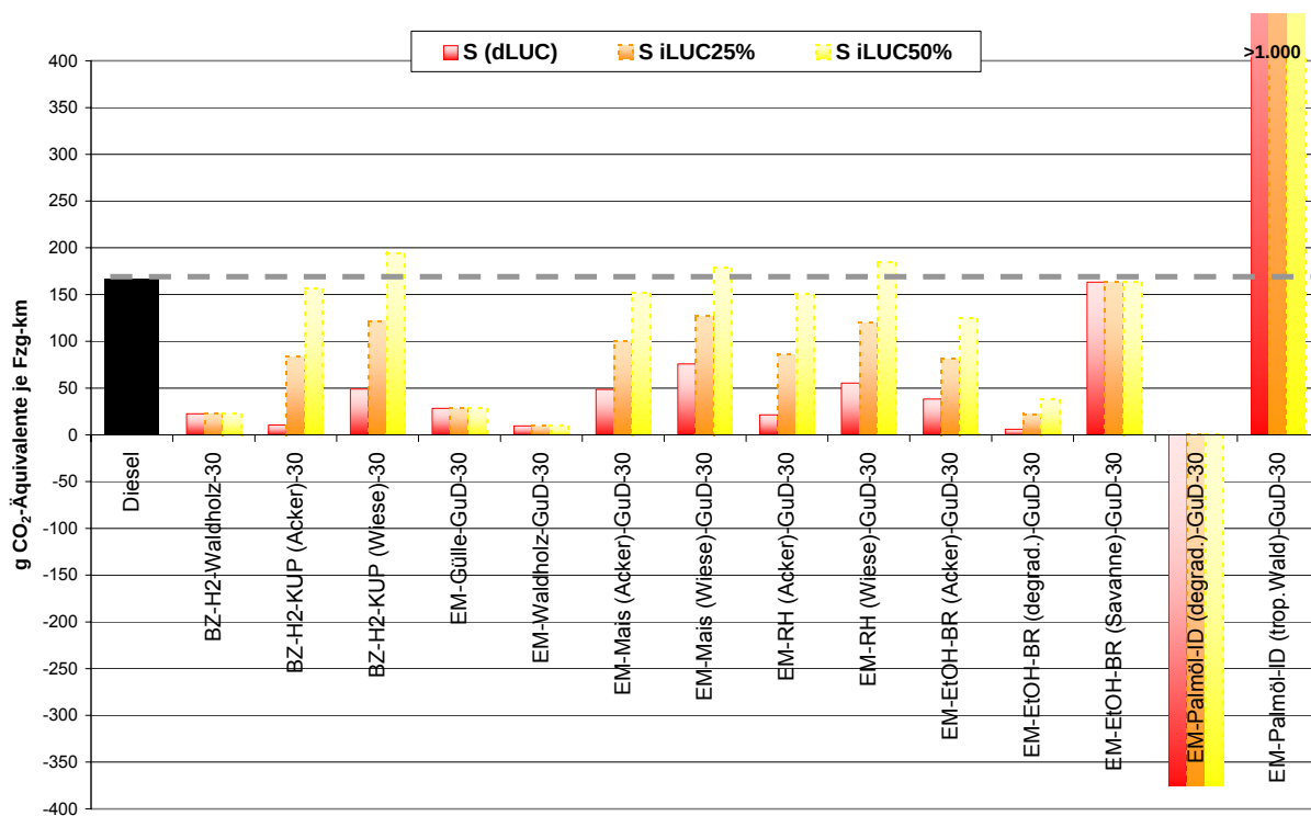
Bild 22 Kumulierte verkehrsleistungsbezogene THG-Emissionen für BioGH 2 und biogenem Fahrstrom
