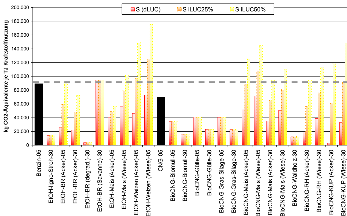
Bild 18 Kumulierte endenergiebezogene THG-Emissionen für Bioethanol und BioCNG
