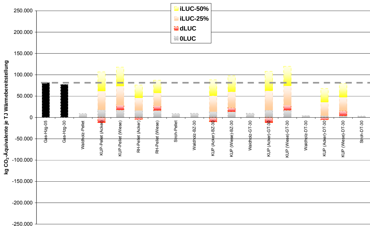
Bild 13 THG-Emissionen der Wärmebereitstellung aus Biomasse
