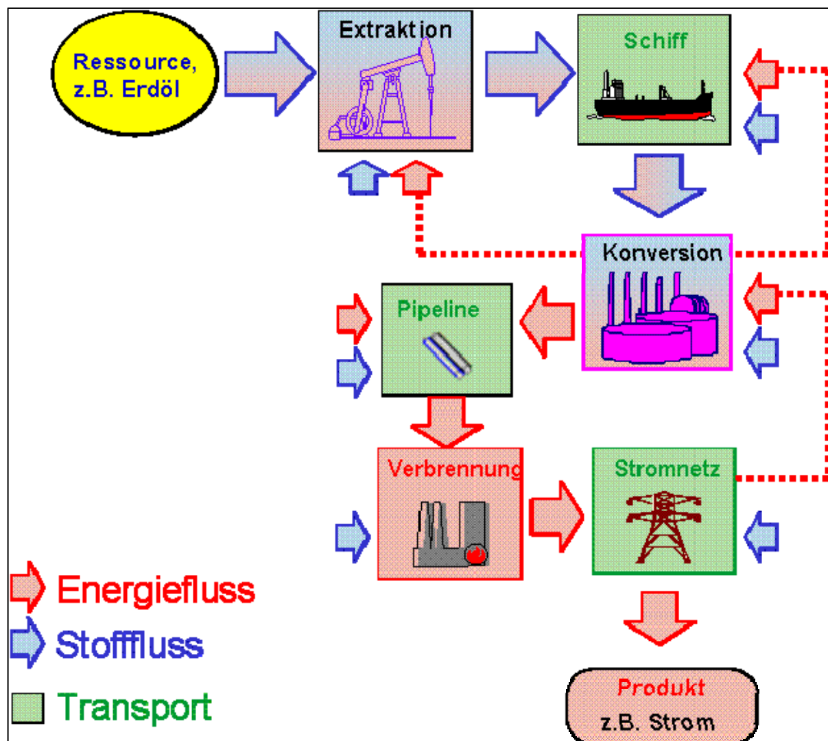
Bild 3 Struktur von Energie- und Stoff-Prozessketten (Vorketten)
