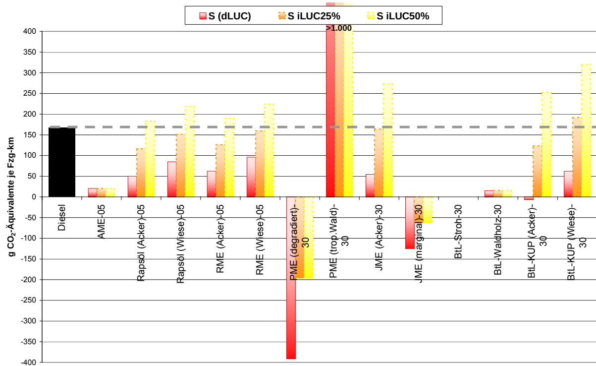
Bild 21 Kumulierte verkehrsleistungsbezogene THG-Emissionen für Biodiesel
