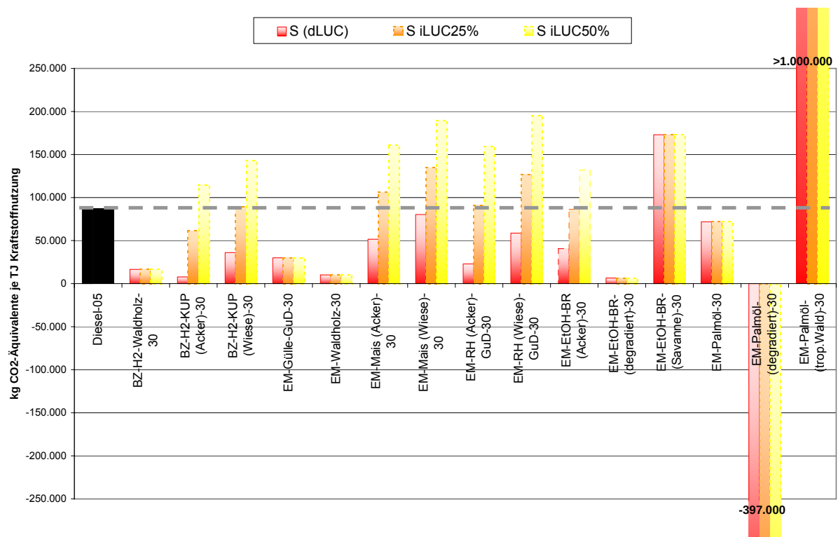
Bild 16 Kumulierte endenergiebezogene THG-Emissionen für Biodiesel sowie BioGH 2 und biogenem Strom
