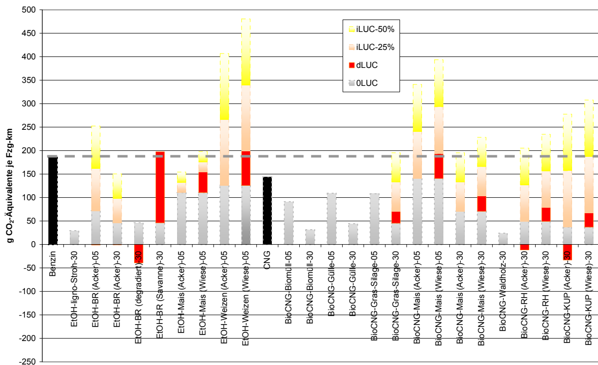
Bild 23 Verkehrsleistungsbezogene THG-Emissionen für Bioethanol und BioCNG
