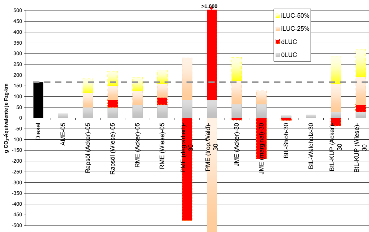
Bild 19 Verkehrsleistungsbezogene THG-Emissionen für Biodiesel
