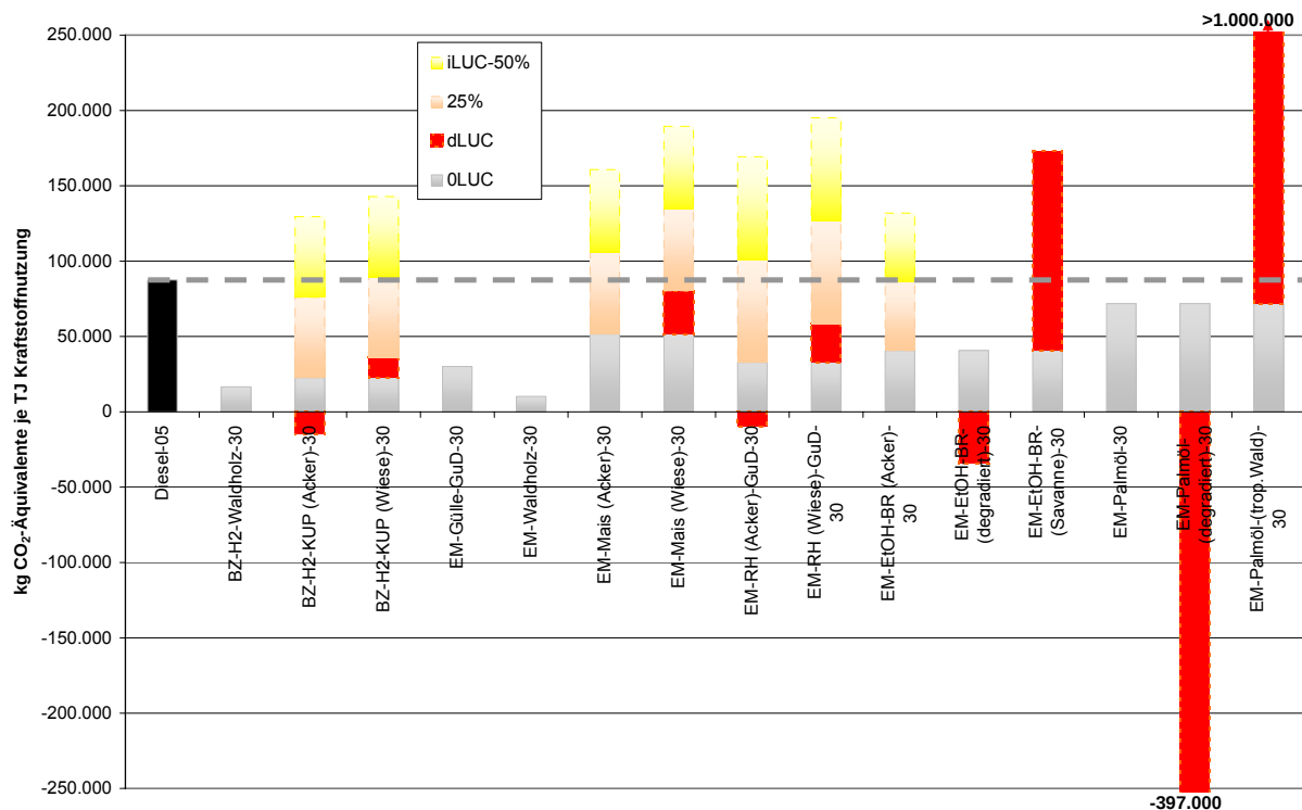
Bild 15 Endenergiebezogene THG-Emissionen für Biodiesel sowie BioGH 2 und biogenem Strom
