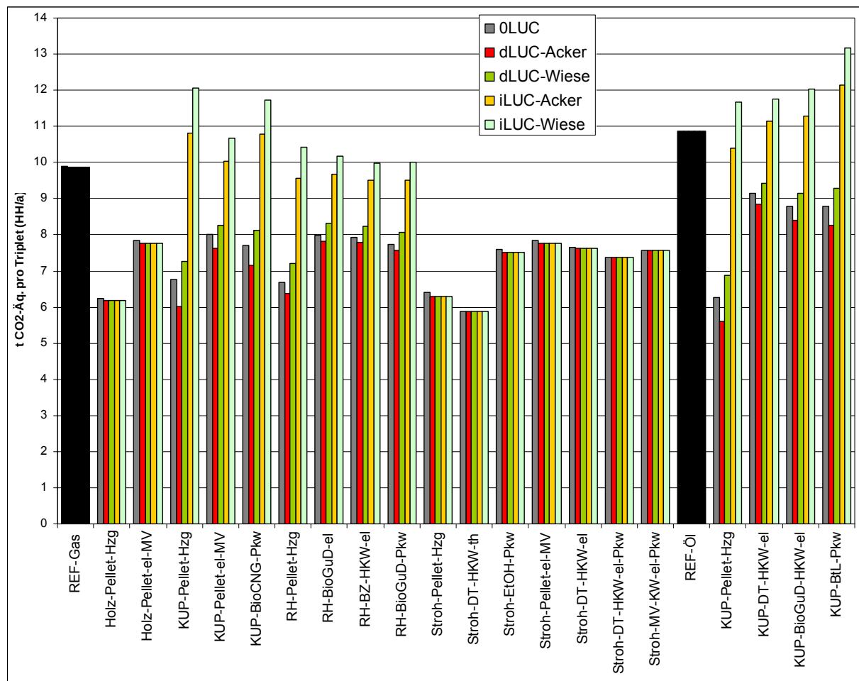
Bild 25 THG-Emissionen für Triplets mit Erdgas/Benzin bzw. Heizöl/Diesel als Referenz sowie biogenen Alternativ-Triplets
