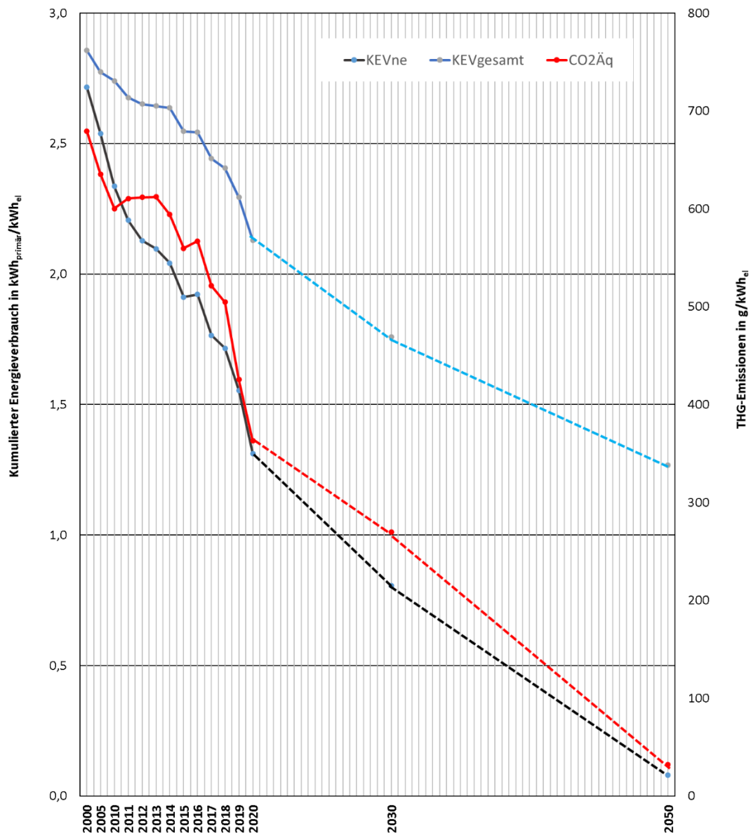
Bild 1 KEV und THG-Emissionen von Strom bei Abgabe aus dem lokalen Netz für 2000 bis 2020 (nach Statistik) sowie 2030 bis 2050 (Szenarien)
