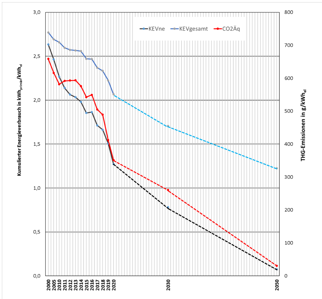
Bild 2 KEV und THG-Emissionen von Strom bei Abgabe aus dem Kraftwerkspark (ohne Netz- und Verteilverluste) für 2000 bis 2020 (nach Statistik) sowie 2030 bis 2050 (Szenarien)
